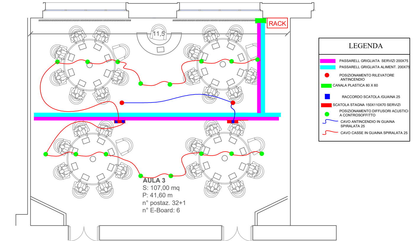
CAVI /TUBAZIONE IMPIANTI SPECIALI LOCALI A SOFFITTO AULA 3 - 1° PIANO
