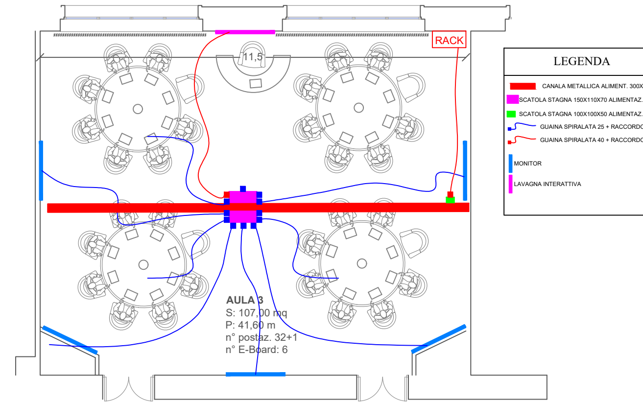
TUBAZIONE PAVIMENTO ALIMENTAZIONE LOCALE AULA 3 - 1° PIANO
