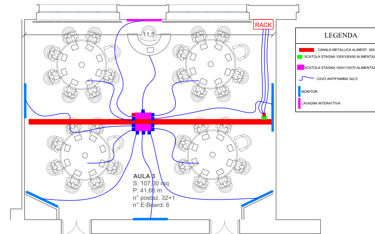
CAVI ALIMENTAZIONE LOCALI A PAVIMENTO AULA 3 - 1° PIANO
