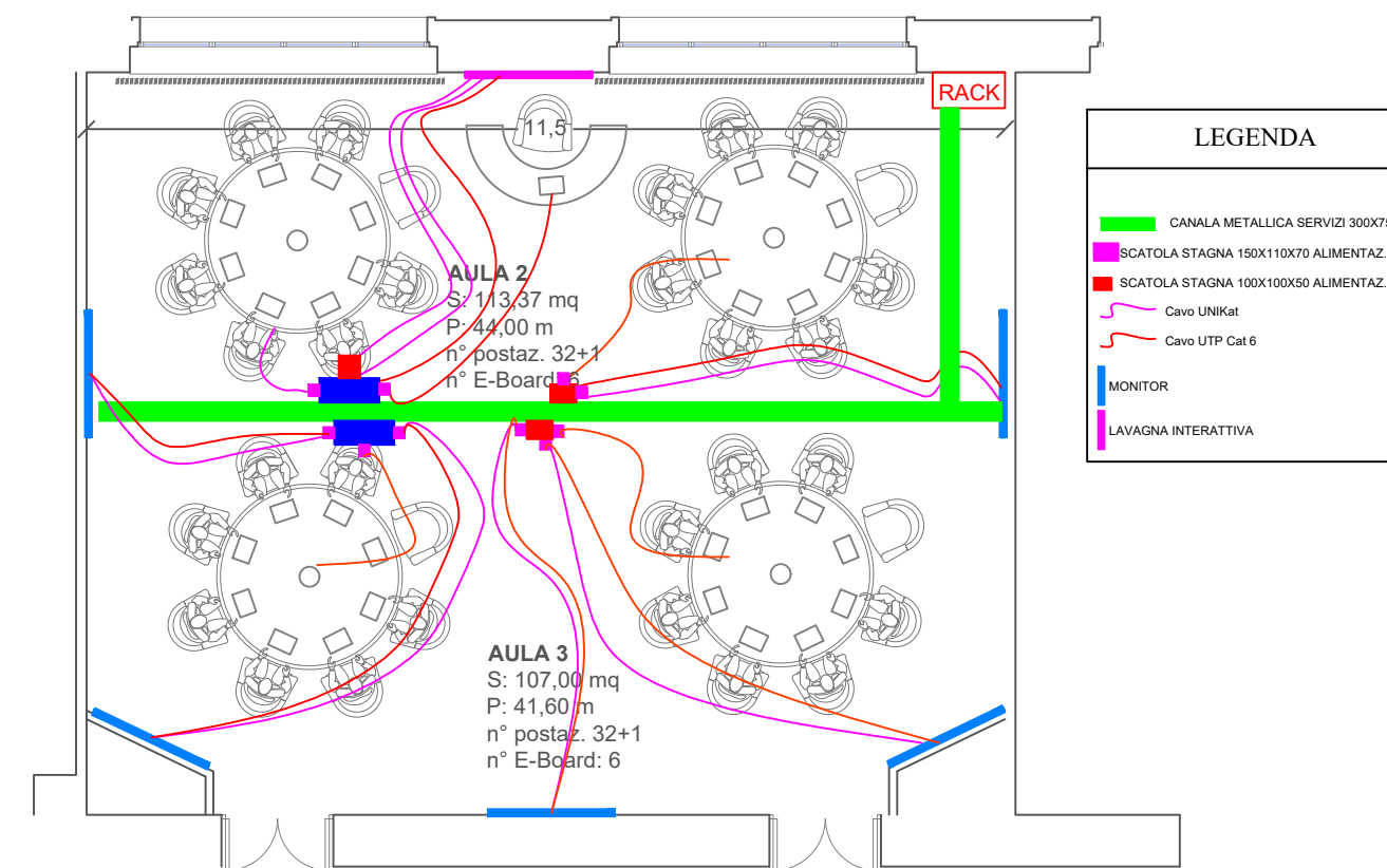
CAVI IMPIANTI SPECIALI LOCALI A PAVIMENTO AULA 3 - 1° PIANO
