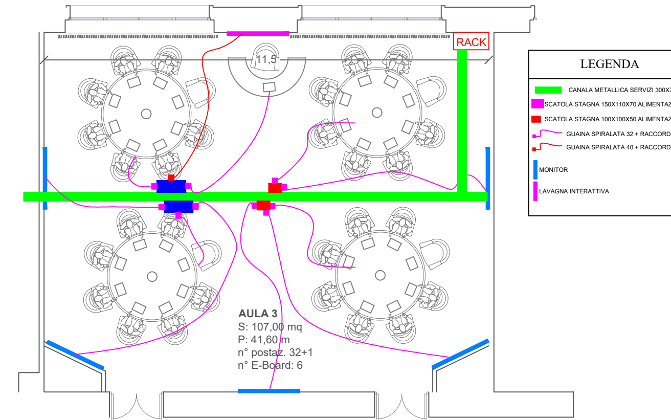
TUBAZIONE PAVIMENTO IMPIANTI SPECIALI LOCALE AULA 3 - 1° PIANO
